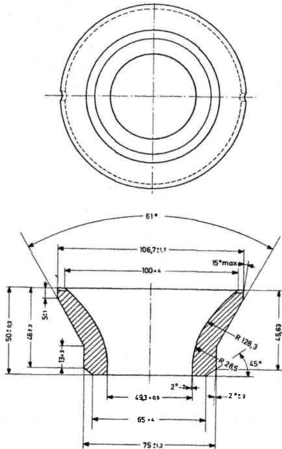
Jochring für 90° Farb-Ablenkeinheiten
