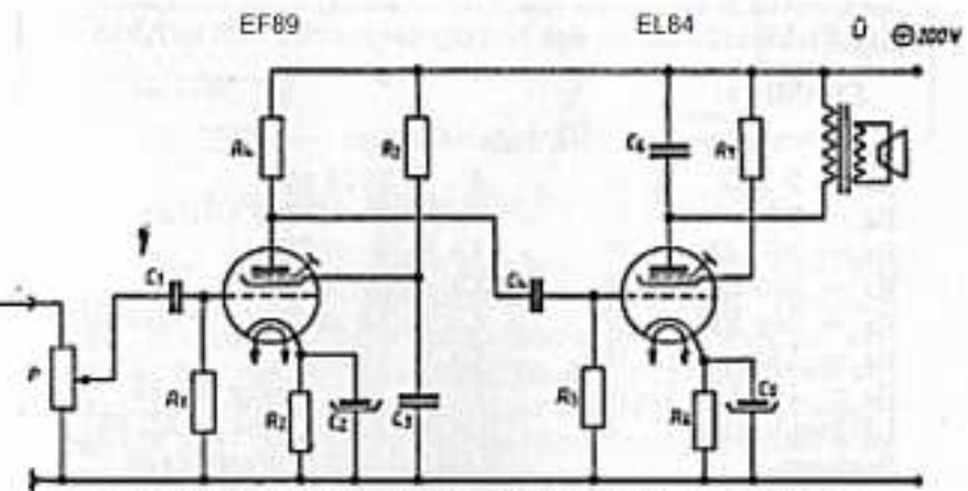
Abb. 36: Schaltung des vollständigen NF-Verstärkers
